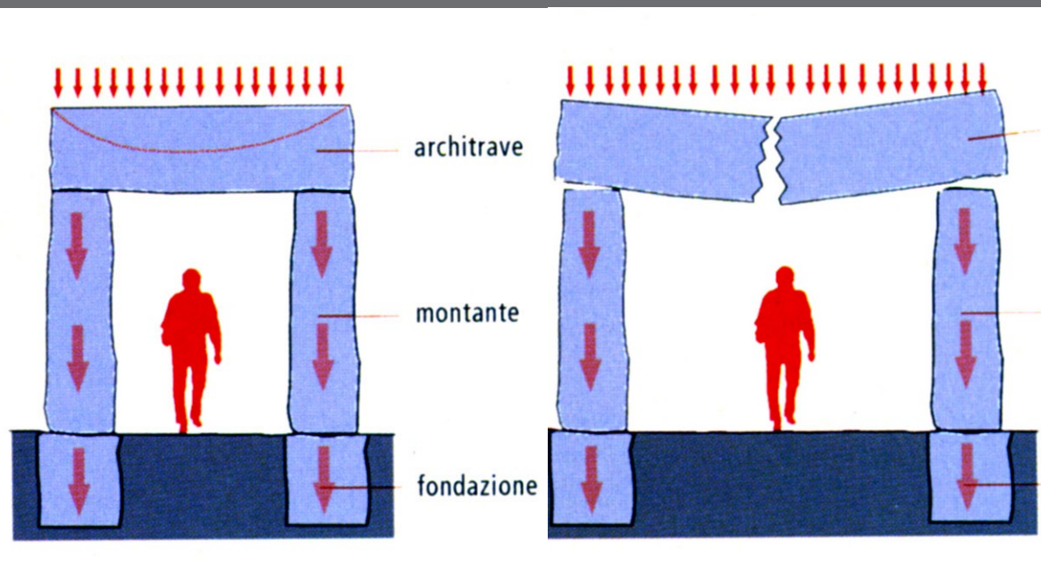
funzionamento e nomenclatura del sistema architravato (o trilitico)
