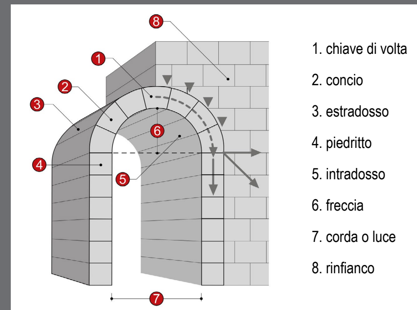
funzionamento e nomenclatura del sistema archivoltato
